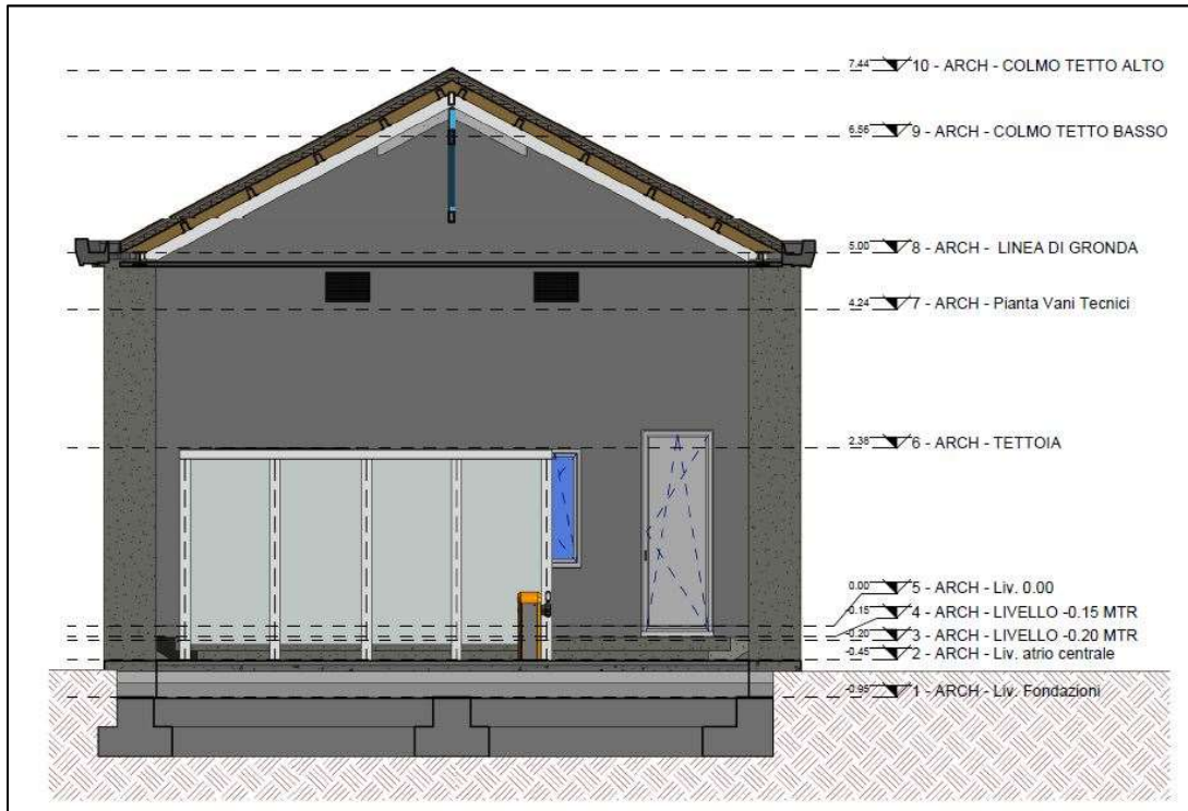
Fig. 3 - Sezione di progetto
