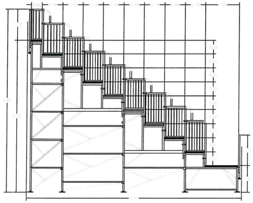
Fig. 3 – prospetto laterale di una tribuna.
